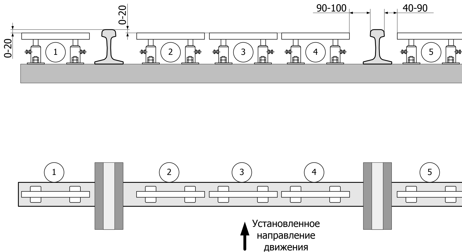
Рисунок А.1 - Габариты установки УКСПС и порядок счета датчиков
